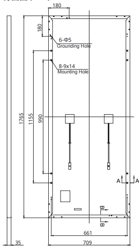
背面図 (mm)
