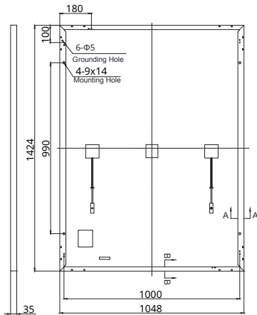
背面図 (mm)
