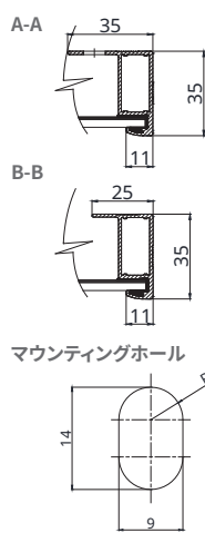
フレーム断面図
