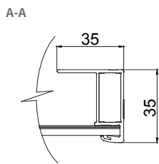
フレーム断面図
