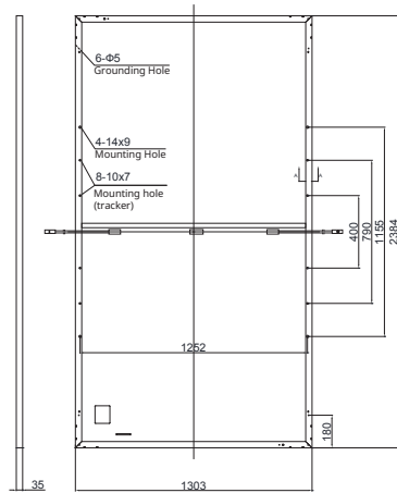
背面図 (mm)
