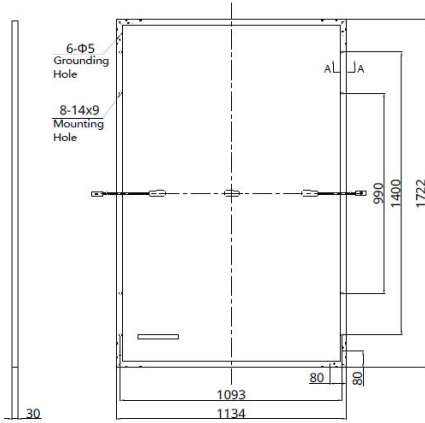
背面図 (mm)
