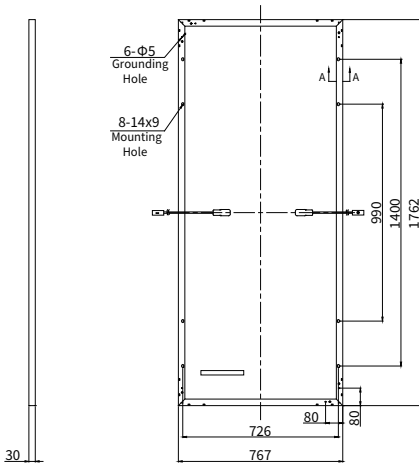
背面図 (mm)
