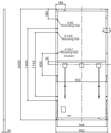
背面図 (mm)
