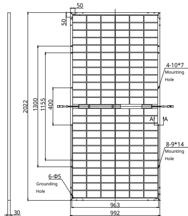
背面図 (mm)
