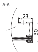
フレーム断面図
