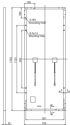
背面図 (mm)
