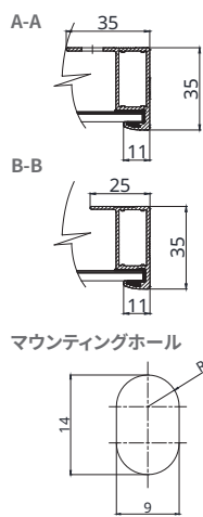
フレーム断面図
