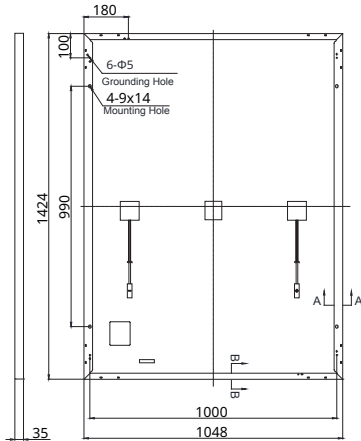
背面図 (mm)
