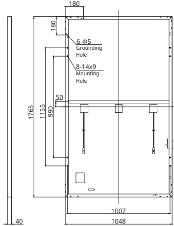
背面図 (mm)
