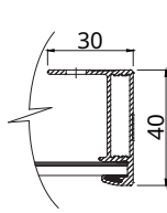
フレーム断面図 A-A
