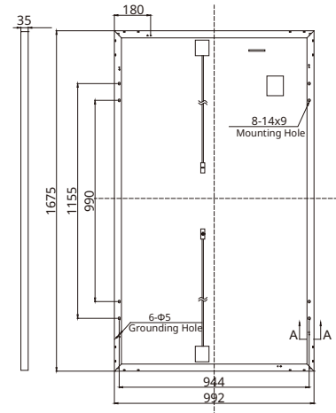
背面図 (mm)
