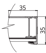
フレーム断面図 A-A
